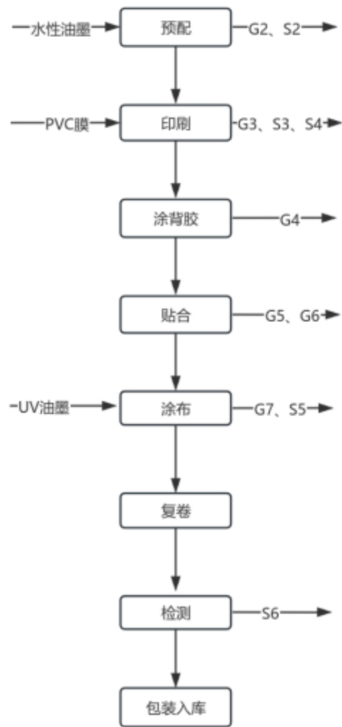
图2-3 水性pvc膜工艺流程及产污环节图
