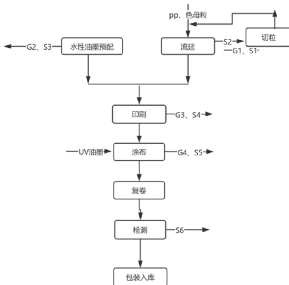
图 2-2 环保 pp 膜工艺流程及产污环节图
