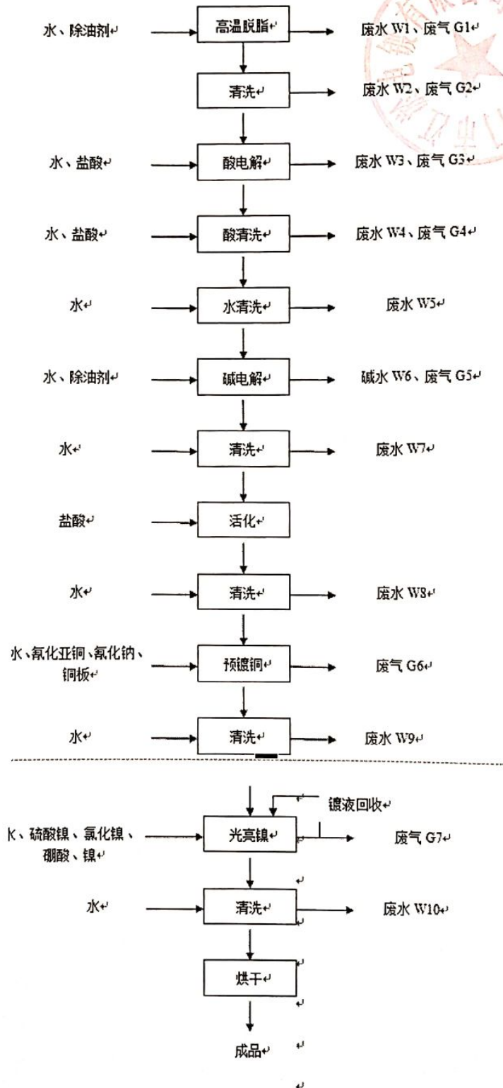
图 3.2-2 自动镀镍件生产工艺流程及产污节点
