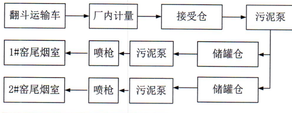
半固态危险废物焚烧系统流程图
