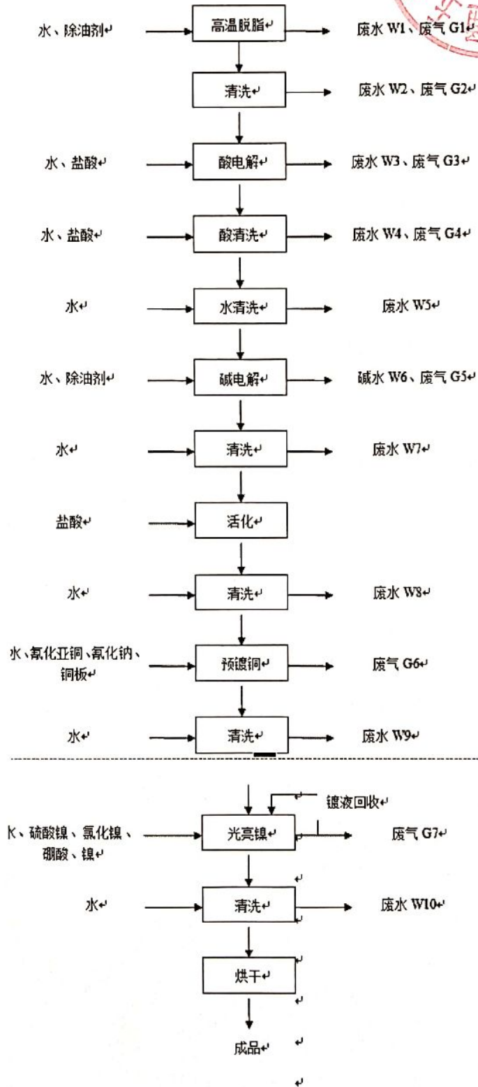
图 3.2-2 自动镀镍件生产工艺流程及产污节点
