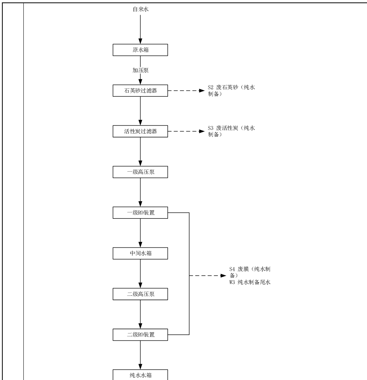
图 2-4 纯水制备工艺流程
