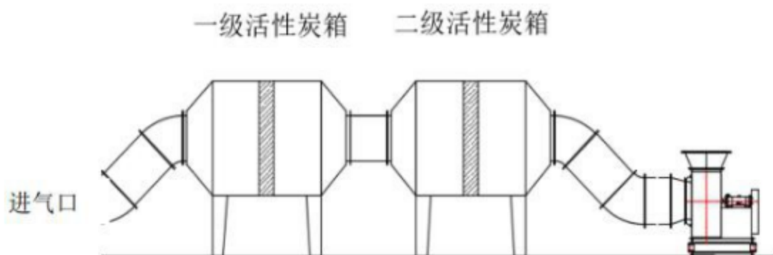
图 4.1-2 二级活性炭吸附装置结构图
