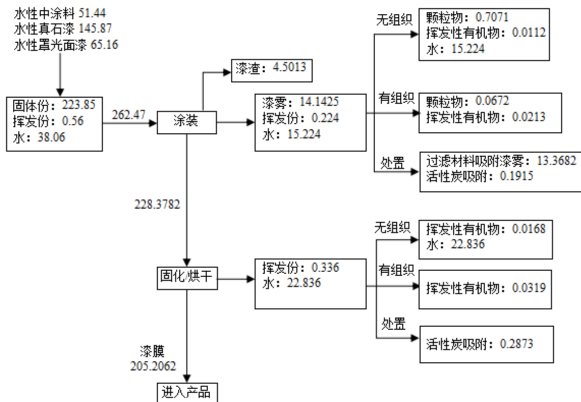
图 2-3 喷漆过程物料平衡图 (单位: t/a)
