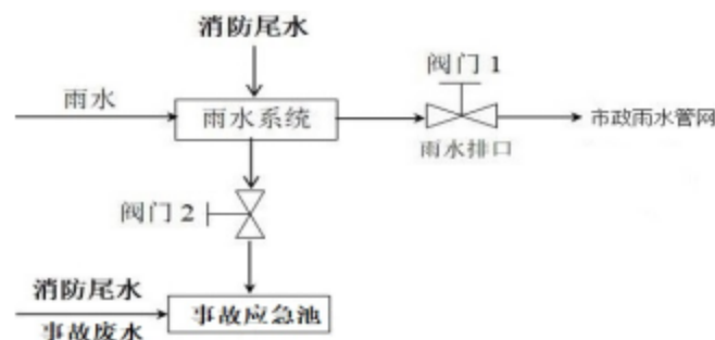
图 4.7-2 事故废水防范和处理流程示意图
