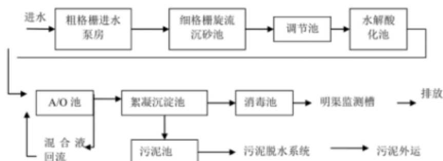
图 4.2-1 南通海川水务有限公司处理工艺流程图
