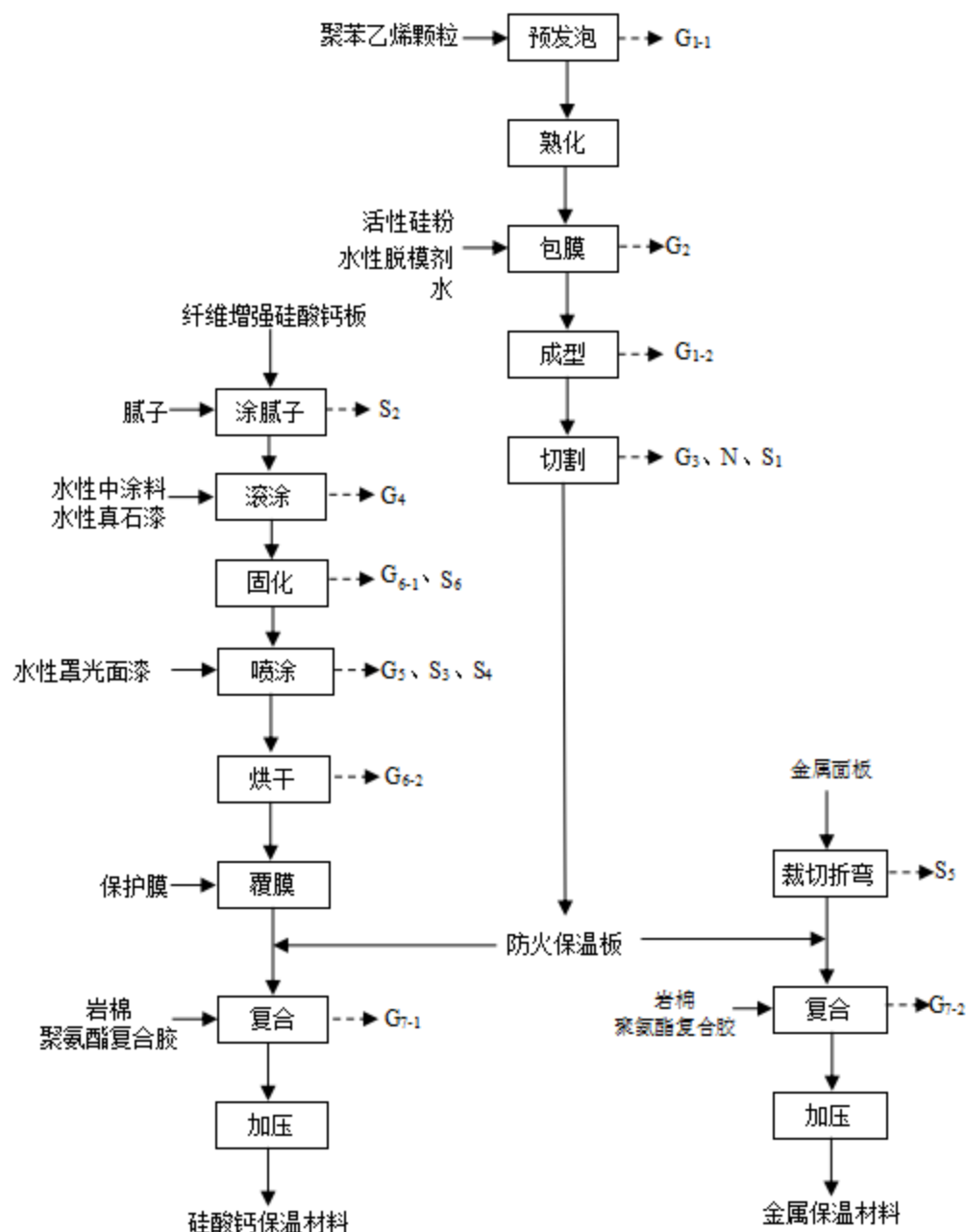
图2-1 生产工艺流程及产物节点图
